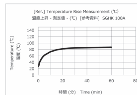
温度上昇 Temperature Rise
