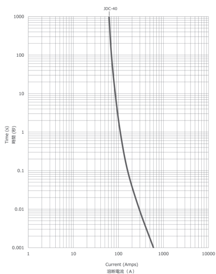
SkyGate DC Fuse JDC-40 (40A) Average Time-Current Curves SkyGate DC ヒューズ JDC-40 (40A) 平均遮断特性曲線
