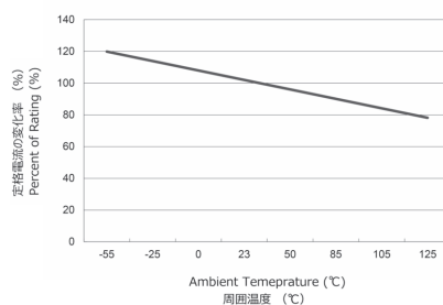
[Ambient Affect Chart on Percent of Rating or Opening Time] 【使用周囲温度 による 定格電流への影響】
