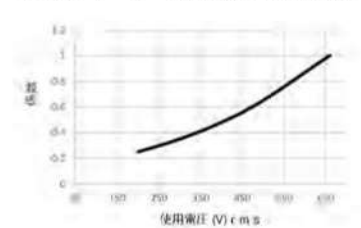
SSF60シリーズ 電圧に対する全遮断 I 2 t
