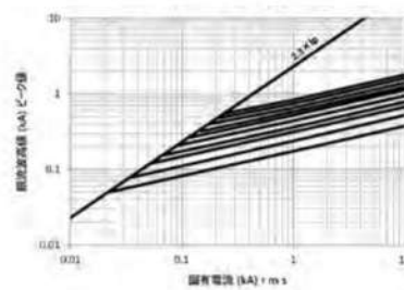
SSF40シリーズ 限流特性
