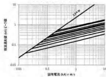
SSF60シリーズ 限流特性
