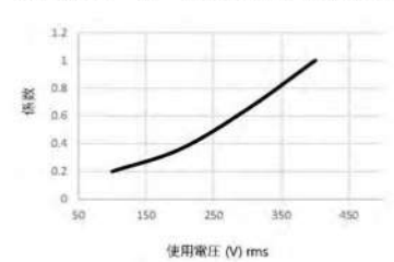
SSF40シリーズ 電圧に対する全遮断 I 2 t
