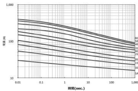
SSF60シリーズ 溶断特性
