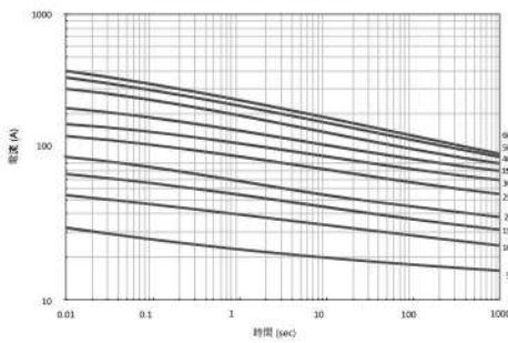
SSF40シリーズ 溶断特性
